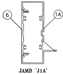
JAMB 'J1A'
